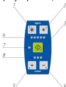
а) с регулировкой цветовой температуры
